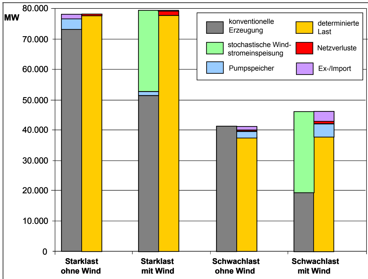
Abbildung 7-9: Gegenüberstellung von Erzeugung, Netzlast, Verlusten und sonstigen Austauschleistungen für die untersuchten Szenarien in 2010
