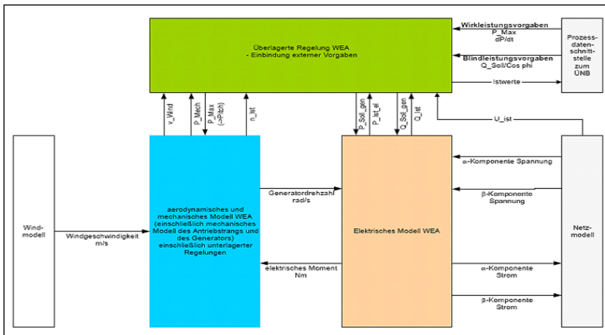
Abbildung 9-2: Übersichtsschaltbild WEA
