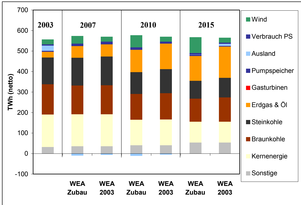
Abbildung 14-9: Stromerzeugung in Deutschland 2003 bis 2015 – Basisszenario + CO 2
