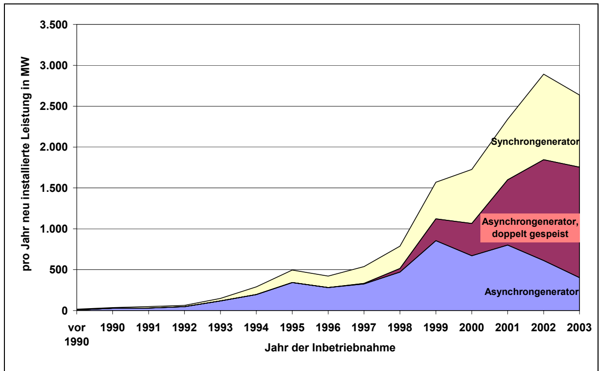
Abbildung 1-5: Entwicklung des jährlichen Windenergiezuwachses in Deutschland nach WEA-Generatortypen
