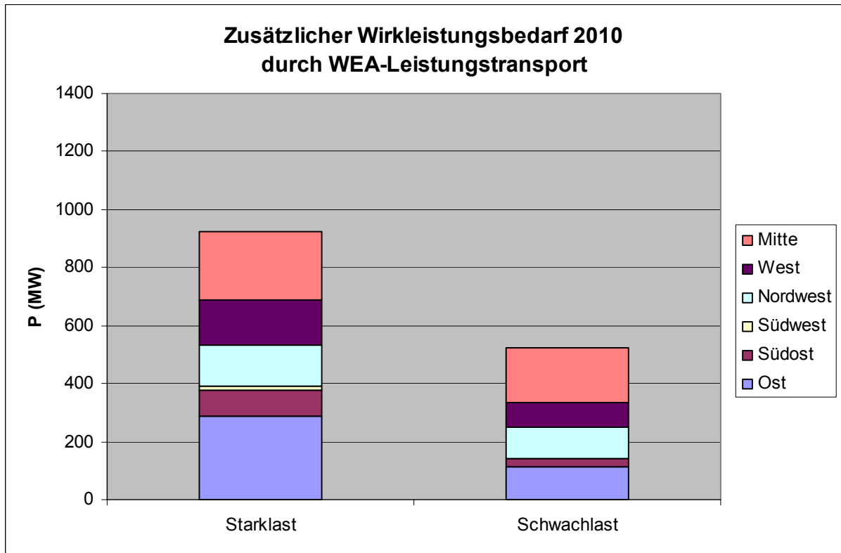
Abbildung 8-9: Zusätzlicher Wirkleistungsbedarf in 2010 bedingt durch den WEA-Leistungstransport
