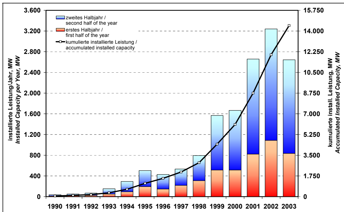
Abbildung 1-1: Entwicklung der jährlich installierten und der kumulierten Windenergieleistung in Deutschland [aus: DEWI (2004)]
