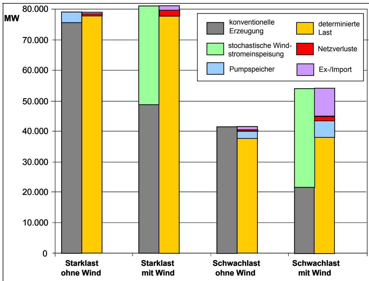
Abbildung 7-12: Gegenüberstellung von Erzeugung, Netzlast, Verlusten und sonstigen Austauschleistungen für die untersuchten Szenarien in 2015
